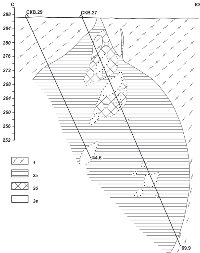
Рис. 3. Увеличение мощности жилы Главной и выклинивание кварц-амазонитовых блоков с глубиной с заменой пегматоидов «матричным» кварц-альбитовым комплексом:
