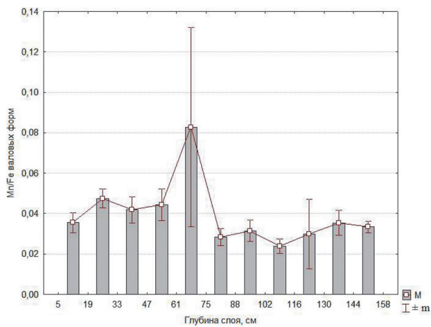
Рис. 3. Изменение отношения валовых и подвижных форм Mn и Fe по профилю донных отложений
