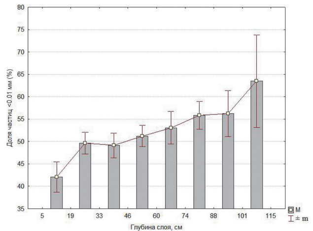
Рис. 5. Изменение содержания частиц <math><0.01 \text{ мм}</math> в донных отложениях с глубиной
