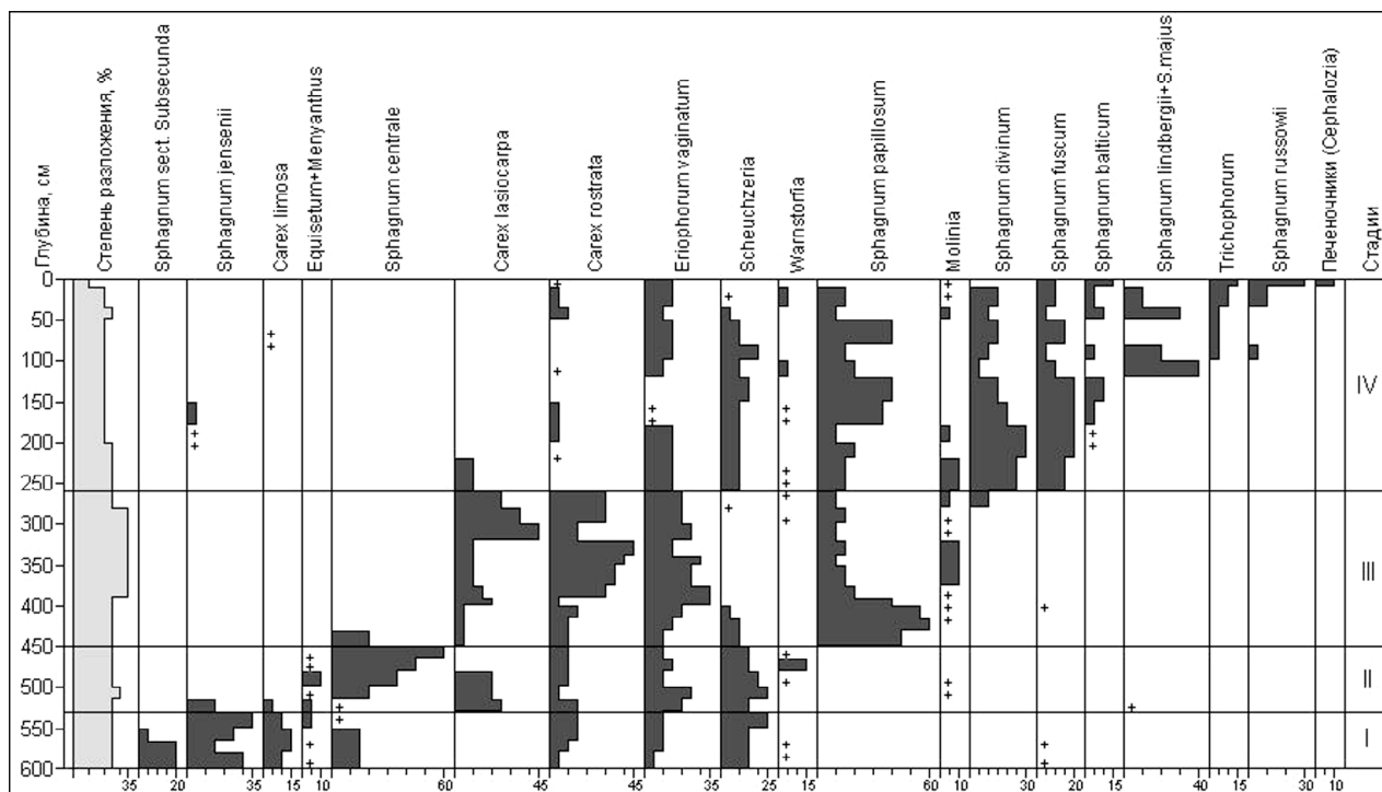
Рис. 6. Диаграмма ботанического состава торфа «висячего» участка на болоте Варгуносу 8 (скв. 6)
